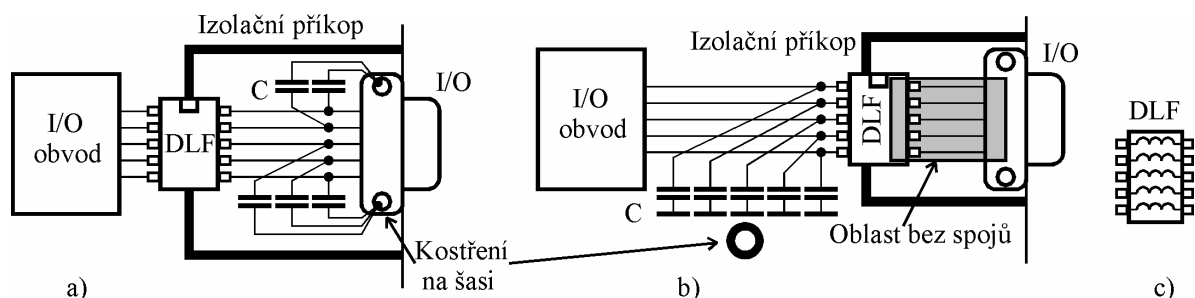
Obr.6.26: I/O filtrace.
