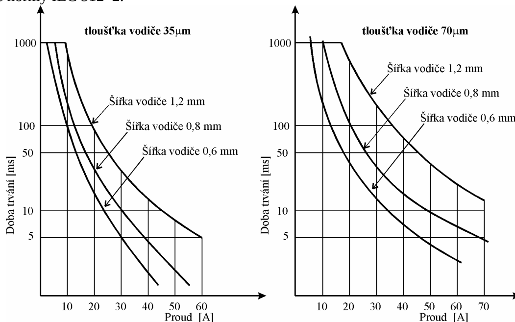
Obr.4.13: Přípustné jednorázové přetížení proudem.
