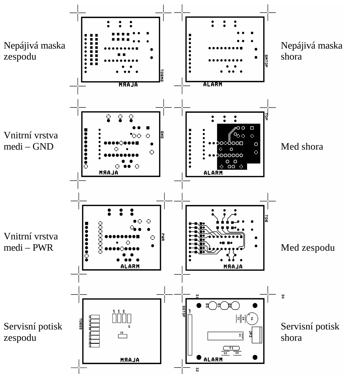
Obr.1.9: Příklad motivu, potřebných pro výrobu čtyrvrstvého plošného spoje s nepájkivou maskou a servisním potiskem (pro výrobní postup podle obrázku 2.4).
