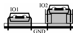
Obr.6.15: Vliv patič.
