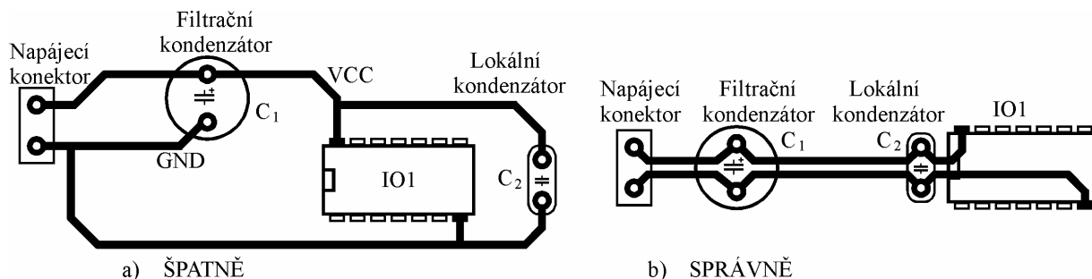
Obr.6.10: Nejčastější chyby při návrhu blokování.
