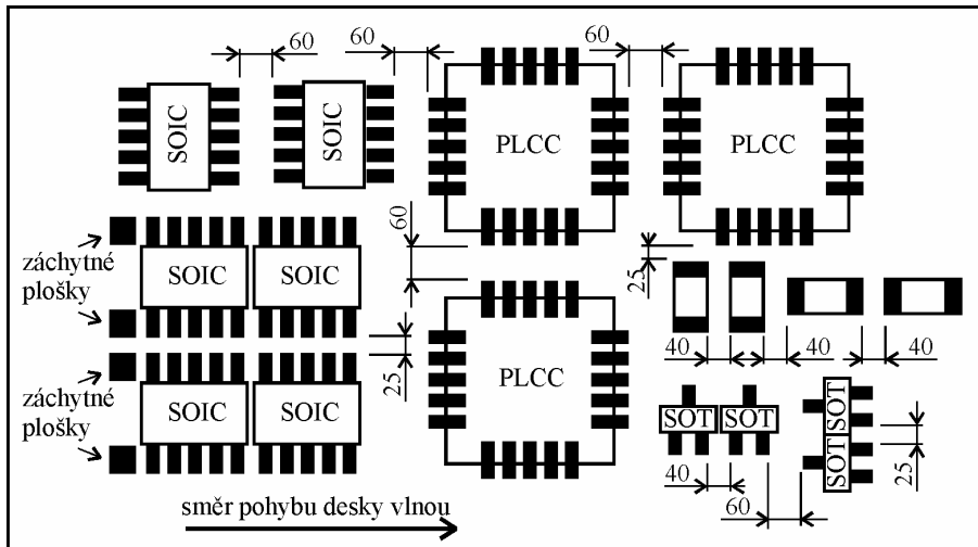
Obr.3.10: Minimální vzdálenosti při různé orientaci součástek [3] (údaje v milech).
