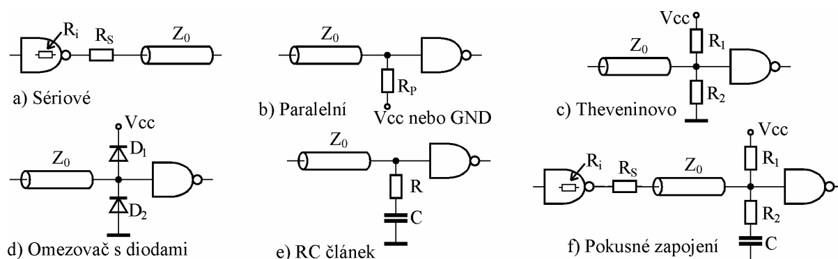
Obr.6.19: Způsoby impedancního prizpusobování.
