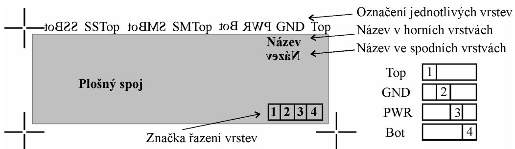
Obr.1.7: Příklad umístění popisu na čtyřvrstvě plošném spoji (pro výrobní postup podle obrázku 2.4).
