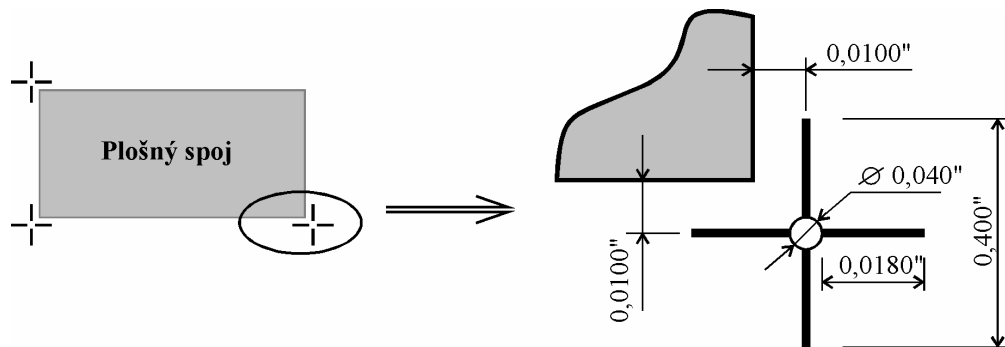
Obr.1.6: Příklad sesazovacích značek a jejich umístění.
