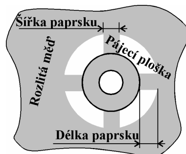
Obr. 1.4: Definice termální plošky.
