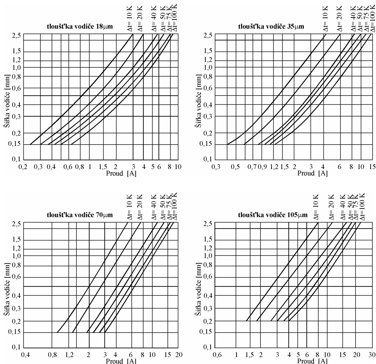
Obr.4.12: Proudová zatížitelnost plošných vodičů (nosný materiál FR4).
