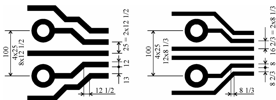
Obr.1.3: Rastr pro 4. a 5. třídu presnosti (rozměry v milech).
