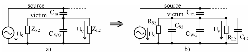
Obr.4.10: Kapacitní vazba.
