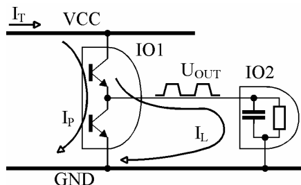
Obr.5.7: Impulzní spotřeba číslicových obvodů.
