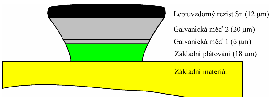
Obr.2.3: Reálný profil leptaného spoje.
