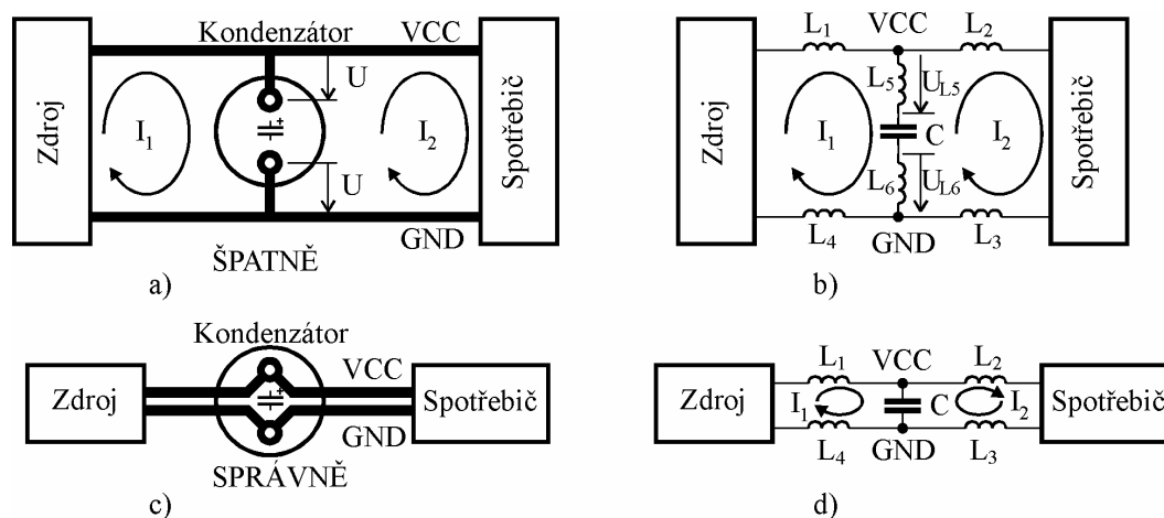
Obr.6.9: Typické problémy umístění blokovacích kondenzátorů.
