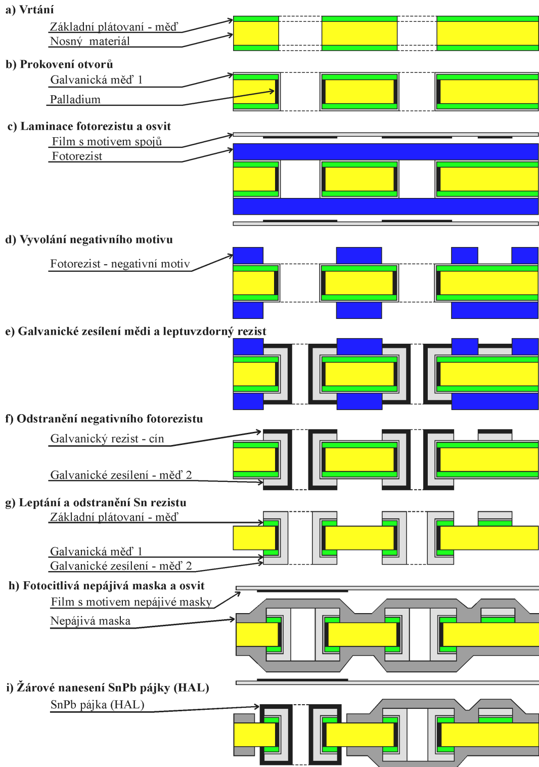
Obr.2.2: Znázornění semiaditivního postupu výroby dvoustranných plošných spoju.
