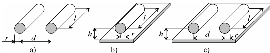
Obr.4.2: Kapacita vodičů kruhového průřezu.
