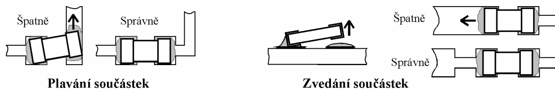
Obr.3.11: Pruvodní jevy při pájení pretavením.
