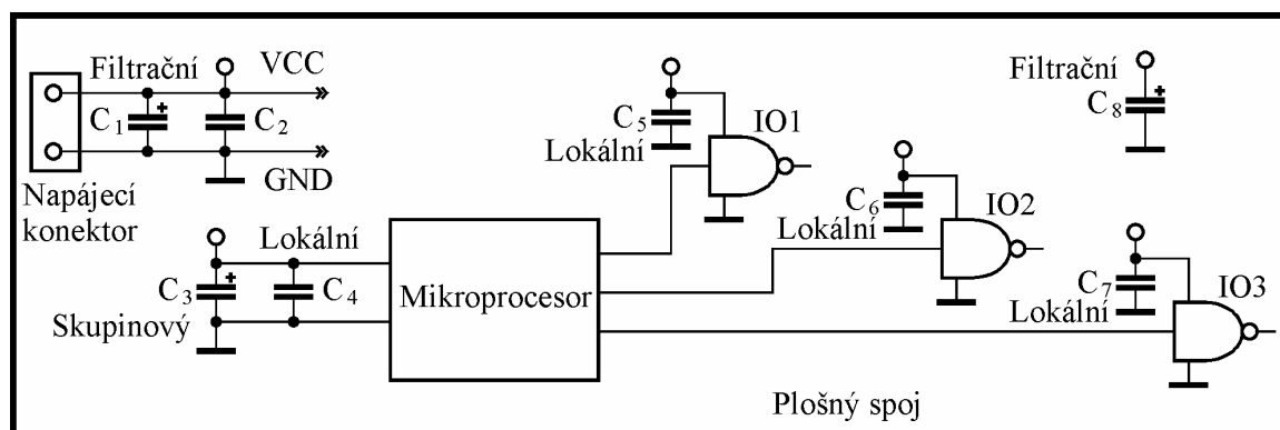
Obr.6.6: Příklad blokování.
