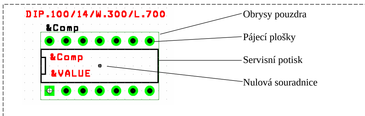
Obr. 1.2: Pouzdro součástky.
