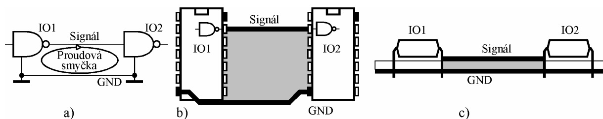
Obr.6.5: Vliv vodivé plochy na velikost proudové smyčky.
