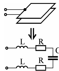
Obr.6.7: Reálný kondenzátor.
